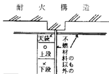
押入等の壁面及び天井面が不燃材料以外の場合
