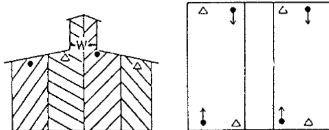
② 越屋根部の幅 (W) 1.5m未満の場合
