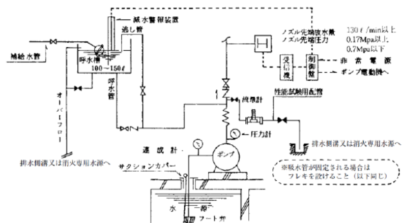
圖 2-2 標準加壓送水裝置例
